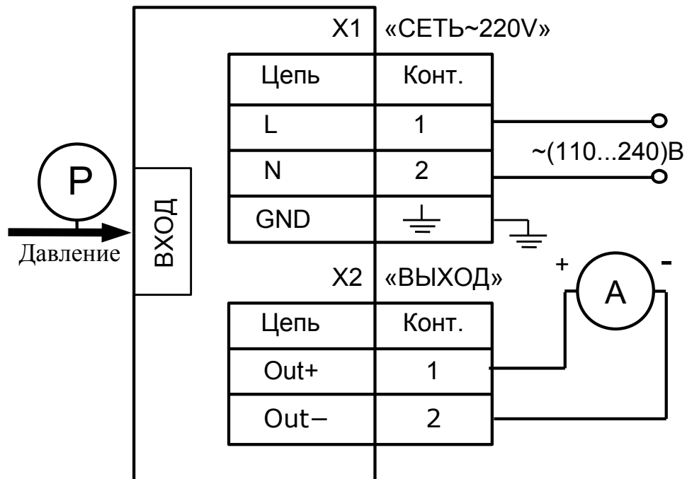
Преобразователь ПЭ-1
